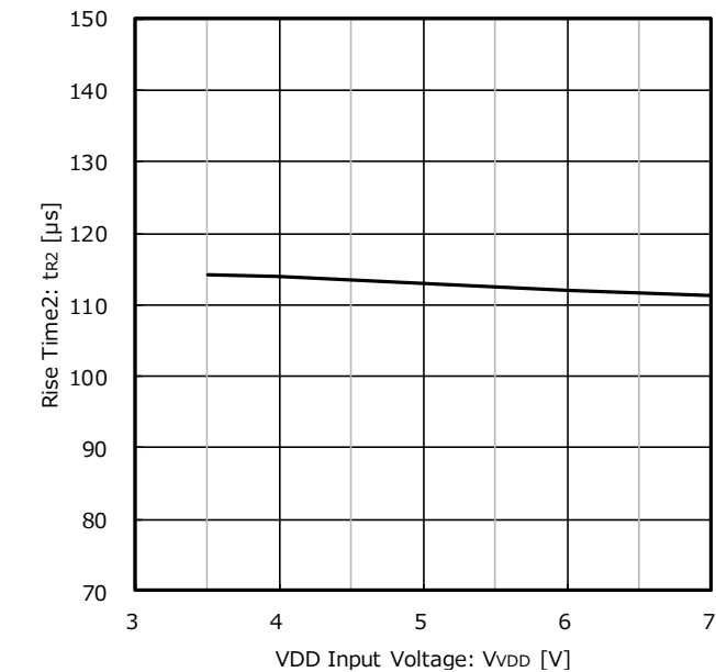
Figure 19. Rise Time2 vs VDD Input Voltage (RSR = 68 kΩ)
