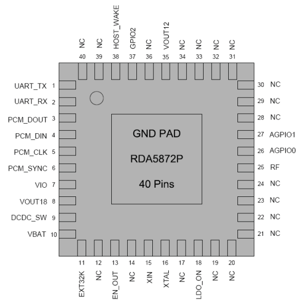
Figure1-1. RDA5872P Top View
