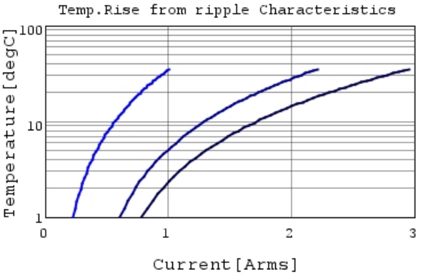
LLL216R71A224MA01 Temp.rise 100kHz
