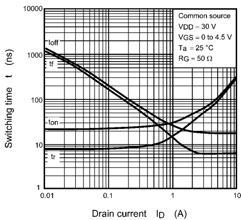
Fig. 8.9 t - I_D
