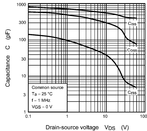
Fig. 8.8 C - V_{DS}
