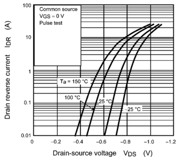
Fig. 8.7 I_{DR} - V_{DS}
