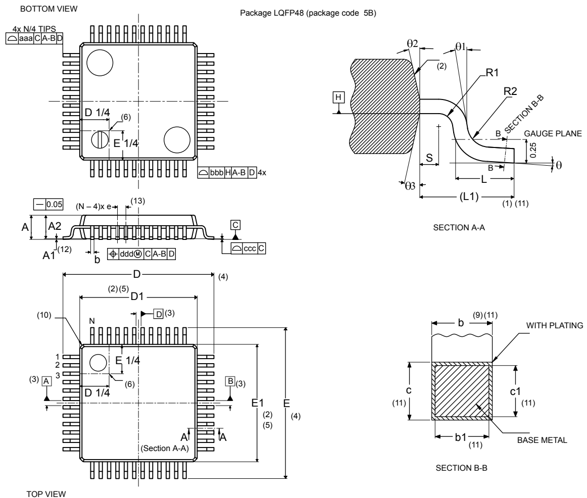
Figure 41. LQFP48- Outline (15.)
