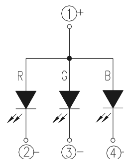
Polarity
