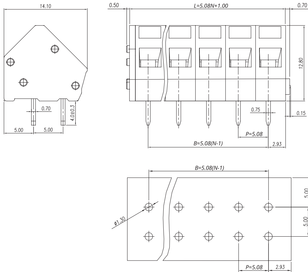
P.C.B. LAYOUT
