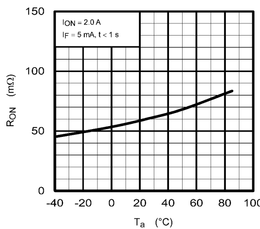
Fig. 16.5 R_{ON} - T_a
