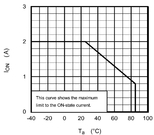
Fig. 16.2 I_{ON} - T_a
