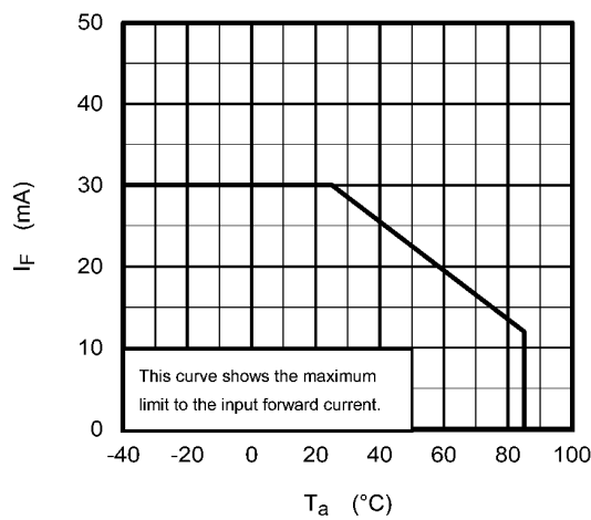
Fig. 16.1 I_F - T_a
