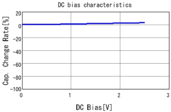
ECASD60E477M009K00 C-DC bias capchange, 25.0degC,
