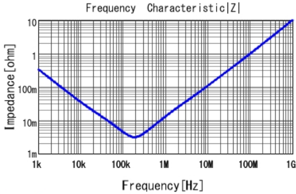
ECASD60E477M009K00 |Z| DC0V, 25degC
