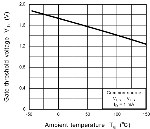
Fig. 8.7 V_{th} - T_a
