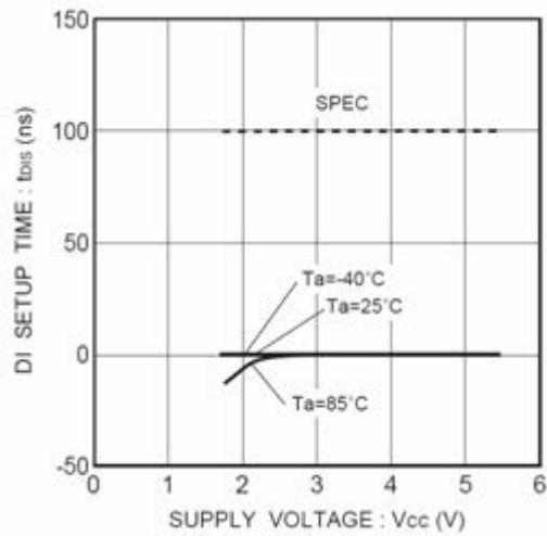
Figure 26. DI setup time t_{DIS}
