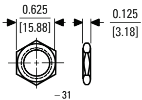
Hex Nut
