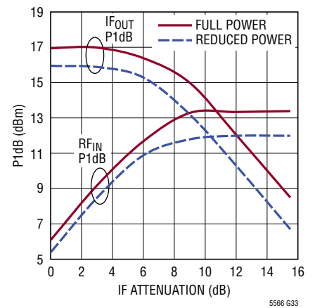
1.9GHz RF Input and IF Output P1dB vs IF Attenuation
