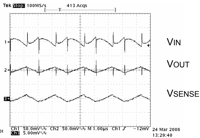
Ripple Noise, V_{IN}=3.3V
