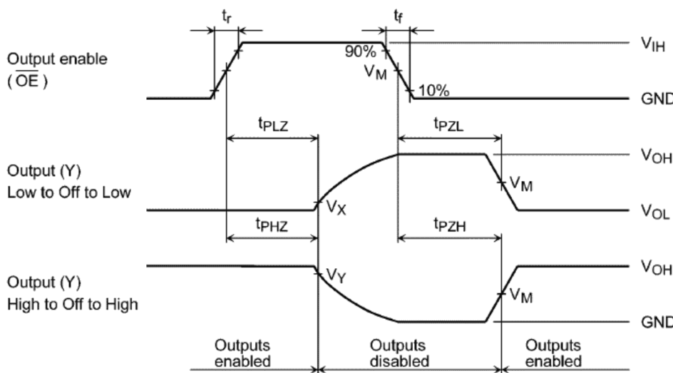
Fig. 12.8.2 t PLZ , t PHZ , t PZL , t PZH
