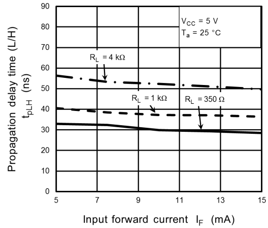
Fig. 12.2.20 t_{pLH} - I_F
