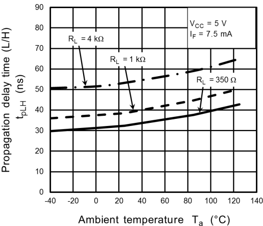
Fig. 12.2.14 t_{pLH} - T_a
