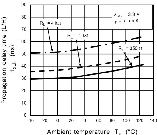
Fig. 12.2.17 t_{pLH} - T_a
