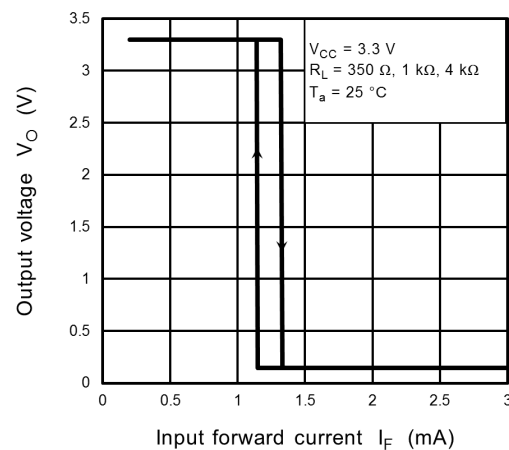
Fig. 12.2.6 V_O - I_F
