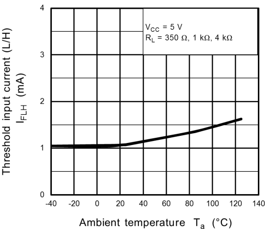
Fig. 12.2.9 I_{FLH} - T_a
