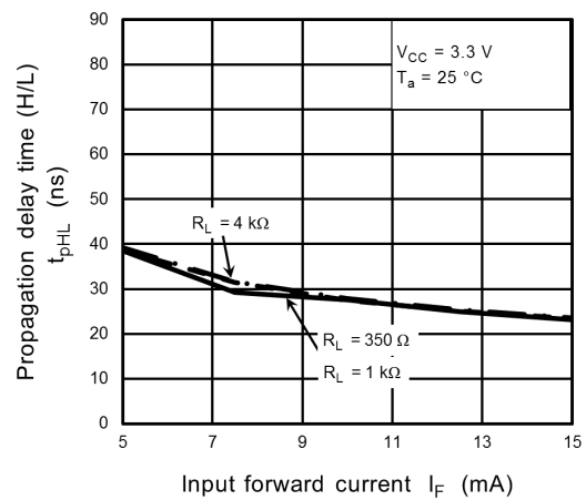
Fig. 12.2.22 t_{pHL} - I_F
