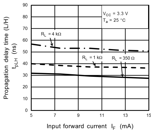
Fig. 12.2.23 t_{pLH} - I_F
