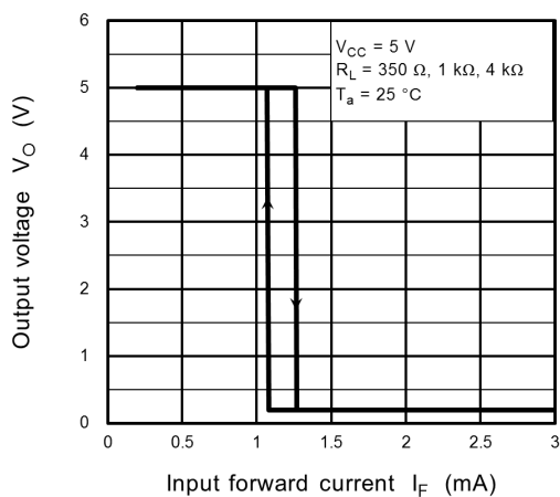
Fig. 12.2.5 V_O - I_F
