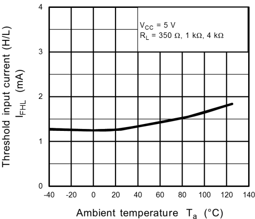
Fig. 12.2.7 I_{FHL} - T_a
