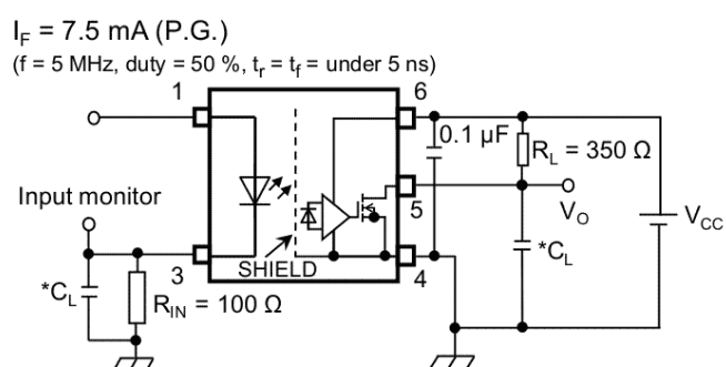
Fig. 12.1.5 I_{FHL} , I_{FLH} , I_{HYS} Test Circuit
