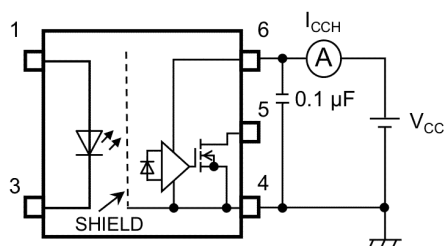
Fig. 12.1.3 I_{CCH} Test Circuit
