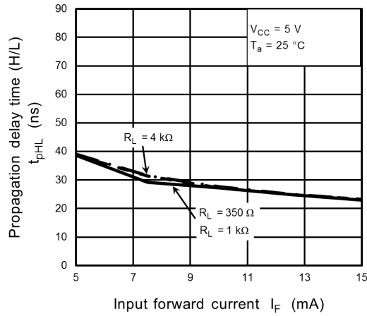
Fig. 12.2.19 t_{pHL} - I_F
