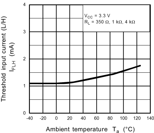
Fig. 12.2.10 I_{FLH} - T_a
