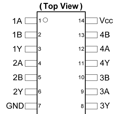
SO-14 / TSSOP-14
