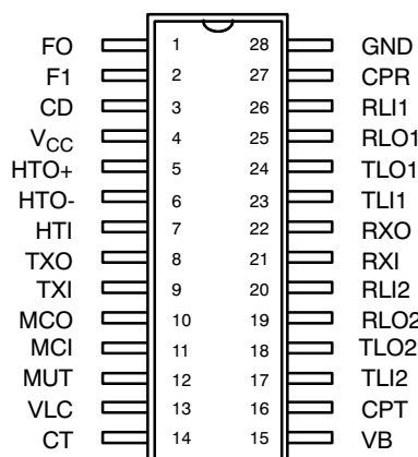
28 Lead Jedec SOIC (300 mil)
