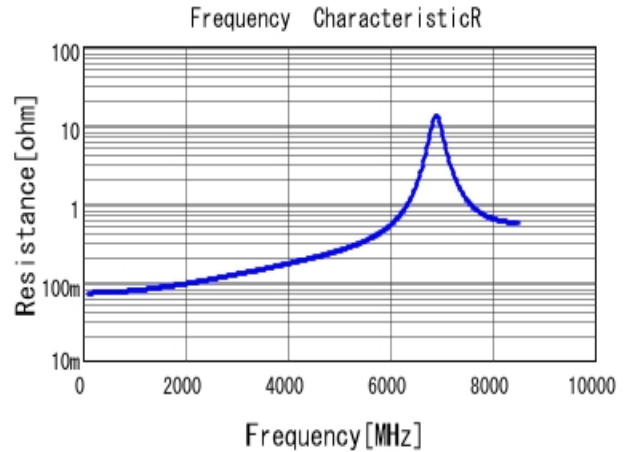
■ GCQ1555C1H9R5DB01 R DC0V, 25degC
