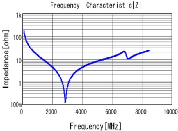
■ GCQ1555C1H9R5DB01 |Z| DC0V, 25degC
