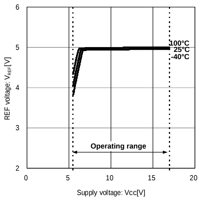
Fig. 4 REF voltage
