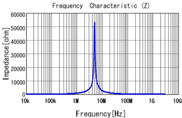
■ MDH6045C-151MB |Z|
