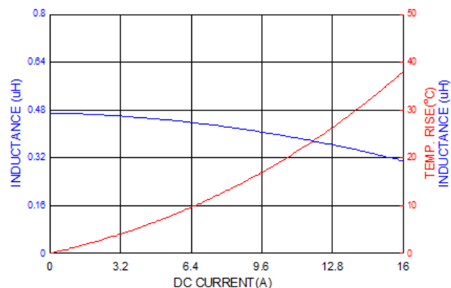
ASPIAIG-FLR4020-R47
