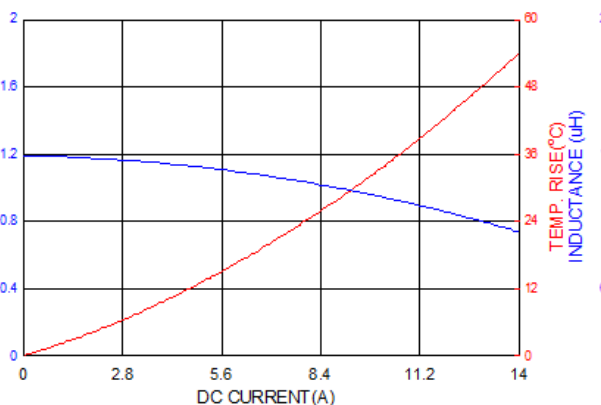
ASPIAIG-FLR4020-1R2
