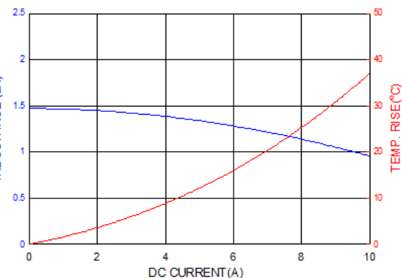
ASPIAIG-FLR4020-1R5
