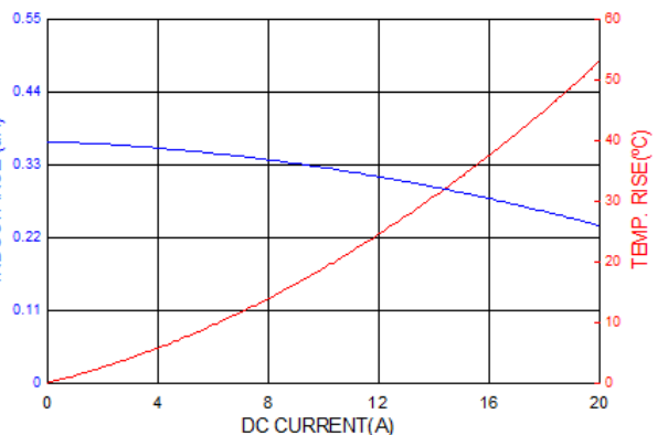
ASPIAIG-F4020-R60
