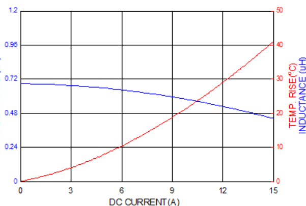
ASPIAIG-FLR4020-R68
