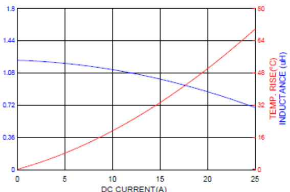
ASPIAIG-F6030-1R2
