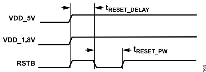
Figure 105. POR Timing
