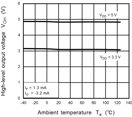
Fig. 12.2.6 V_{OH} - T_a
