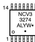
TSSOP-14 DTB SUFFIX CASE 948G
