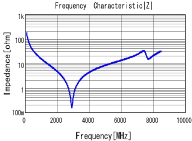
■ GCQ1555C1H9R1DB01 |Z| DC0V, 25degC
