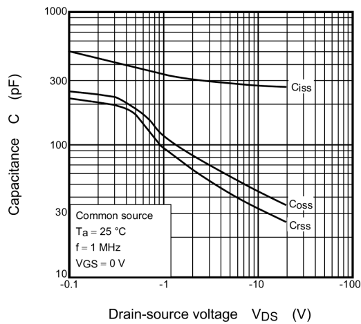
Fig. 8.9 C - V_{DS}
