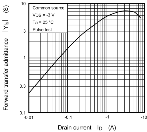
Fig. 8.7 |Y_{fs}| - I_D
