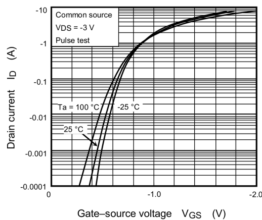
Fig. 8.2 I_D - V_{GS}
