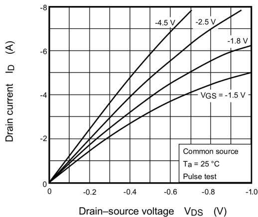
Fig. 8.1 I_D - V_{DS}
