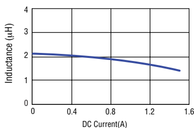
SRN2010TA-2R2M
