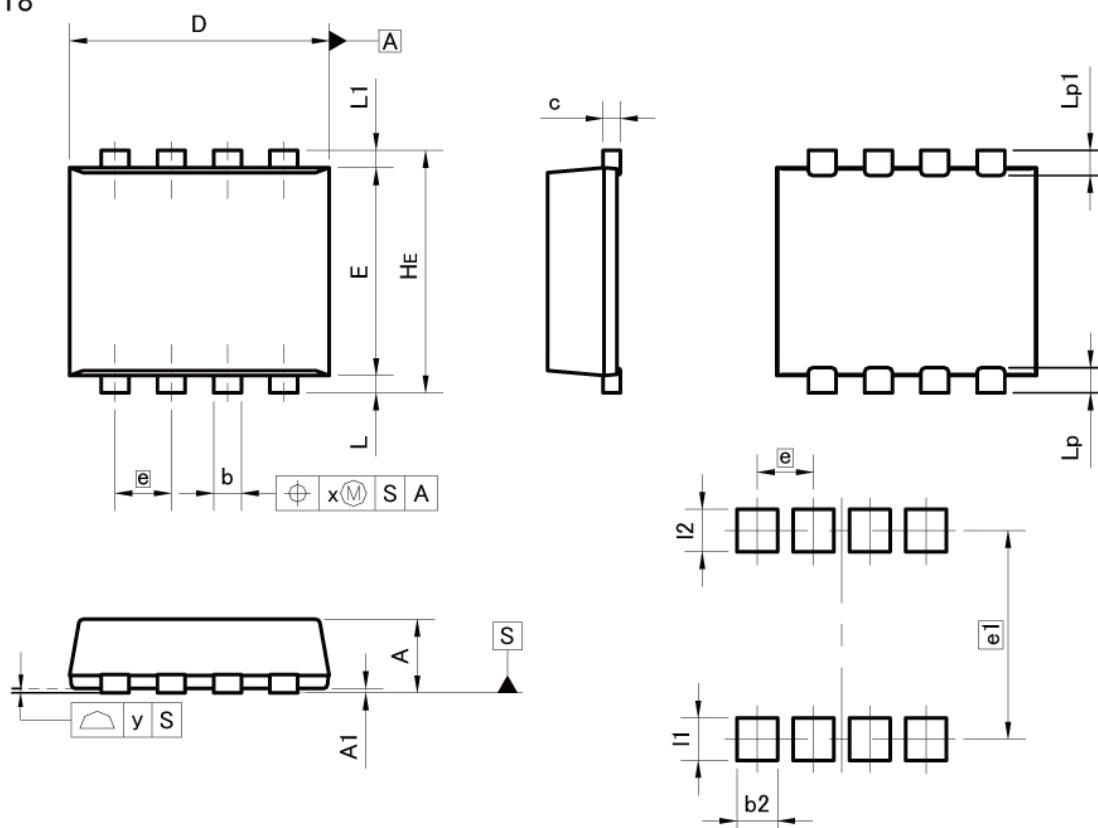
TSMT8
