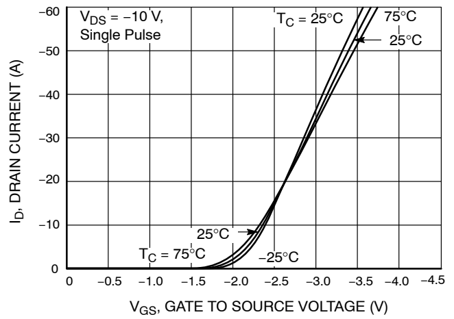
Figure 3. I_D - V_{GS}
