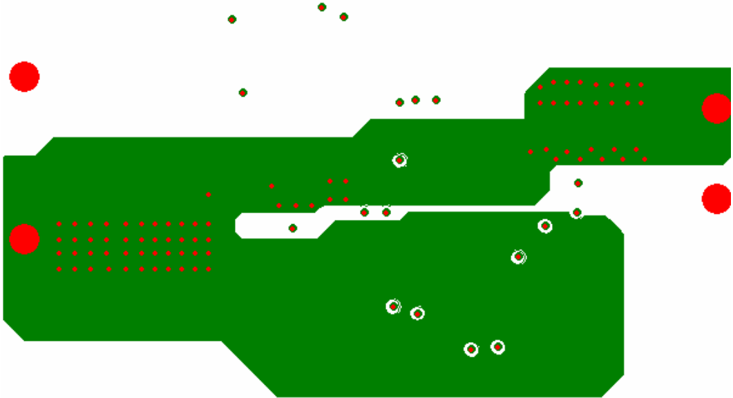
Internal Layer 3
