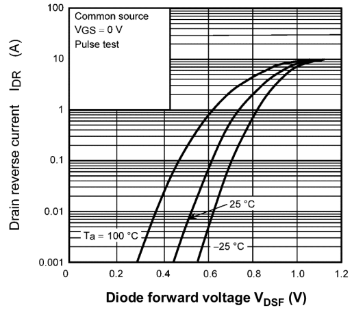
Fig. 8.8 I_{DR} - V_{DSF}
