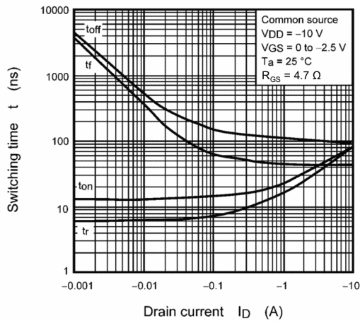
Fig. 8.11 t - I_D
