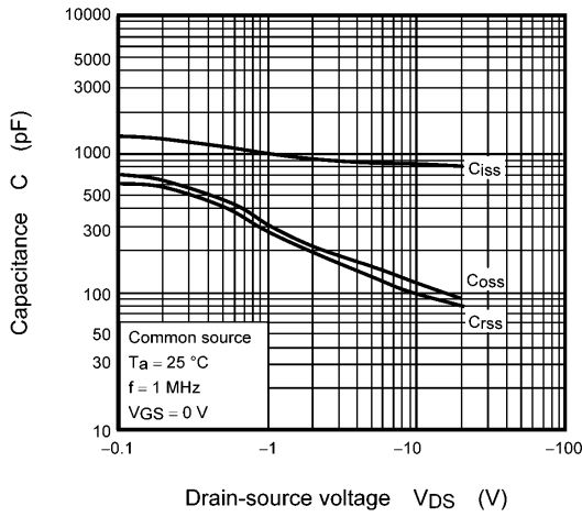
Fig. 8.9 C - V_{DS}
