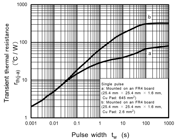
Fig. 8.12 r_{th(j-a)} - t_w
