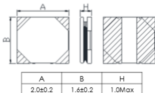
Dimension (Unit:mm)
