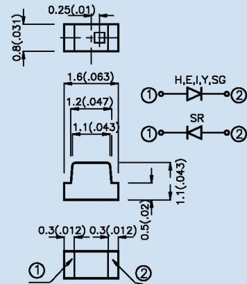
1.6 mm x 0.8 mm (0603)
