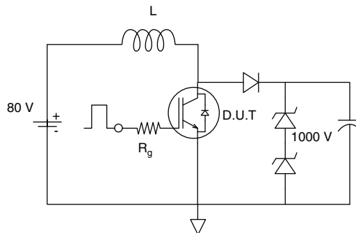
Fig. 26 - RBSOA Circuit
