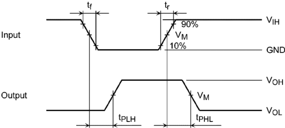
Fig. 11.8.1 T PLH , T PHL
