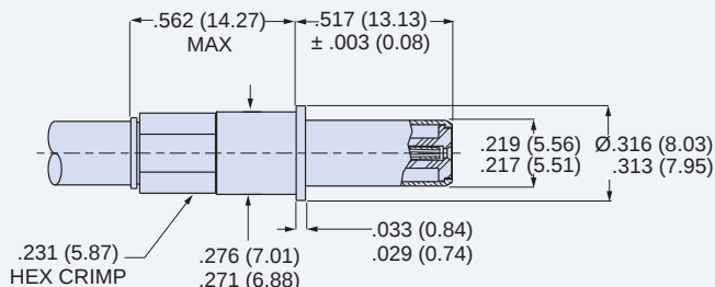
Socket Contact 852-083
