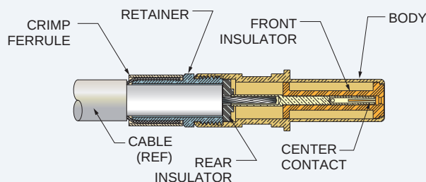
Socket Contact 852-083
