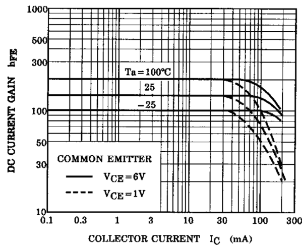
Fig. 8.2 h_{FE} - I_C
