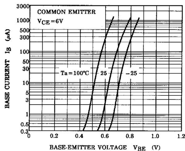
Fig. 8.6 I_B - V_{BE}
