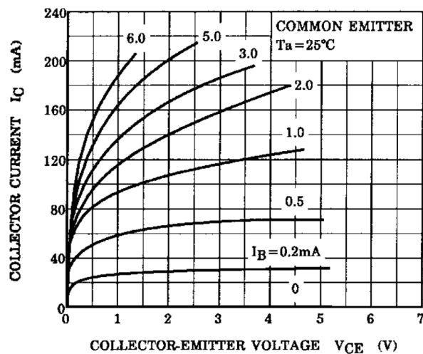
Fig. 8.1 I_C - V_{CE}
