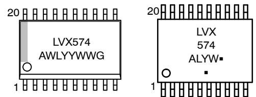
SOIC-20
