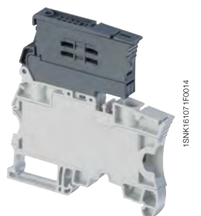
ZS10-SF
