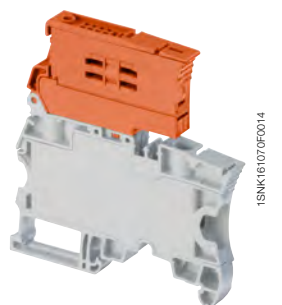
ZS10-S-R2
