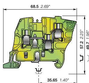
ZS6-3S-PE
