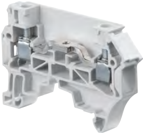
ZS4-R1
