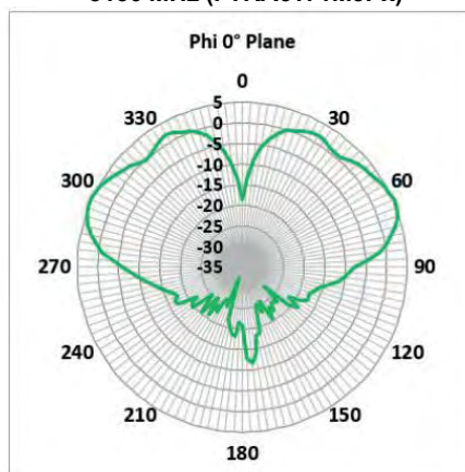
5150 MHz (FTRA6171M5Px)
