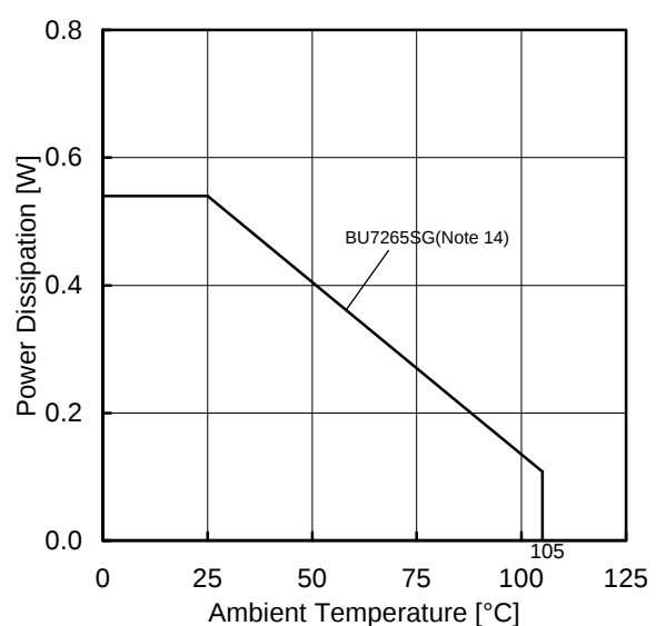
(d)BU7265SG
