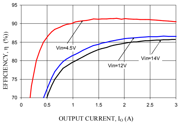
V_o = 1.8V
