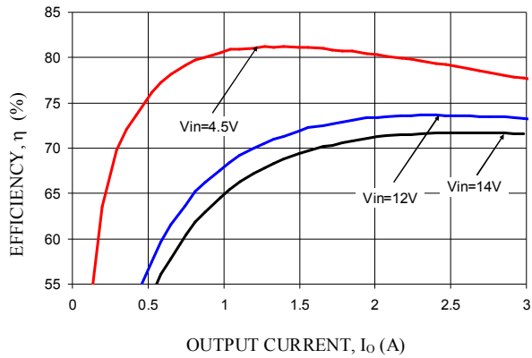
V_o = 0.6V
