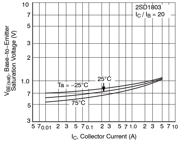
Figure 16. V_{BE(sat)} - I_C
