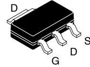
SOT-223 CASE 318H-01
