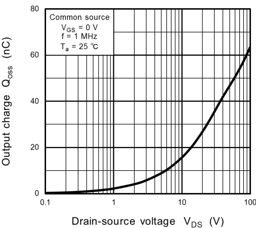
Fig. 8.12 Q_{oss} - V_{DS}
