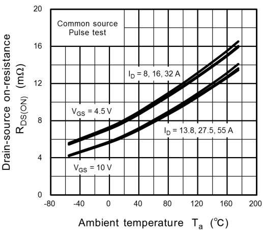
Fig. 8.9 R_{DS(ON)} - T_a
