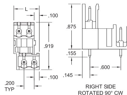
ELFD—Vertical
