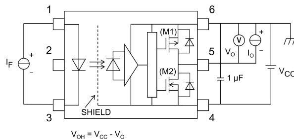
Fig. 13.1.3 VOH Test Circuit
