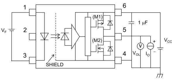
Fig. 13.1.4 VOL Test Circuit
