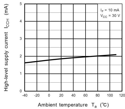
Fig. 13.2.6 I_{CCH} - T_a
