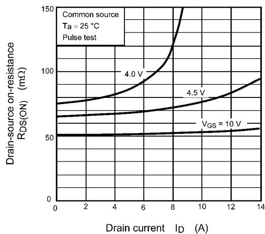
Fig. 8.2 R_{DS(ON)} - I_D
