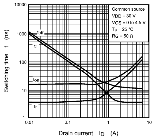
Fig. 8.4 t - I_D
