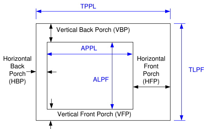
Figure 10-1. Parameter Definitions
